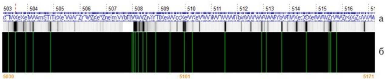
Рис. 2. Сравнение спектрограмм атома никеля, экспериментально полученной (а) и эмулированной из ЭСА (б) в видимой области (5030-5171) Å.
